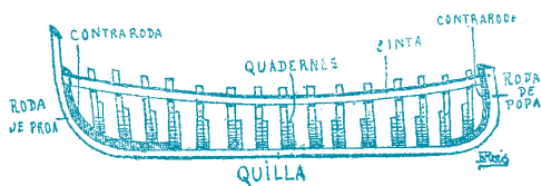
Parts essencials d'una barca
